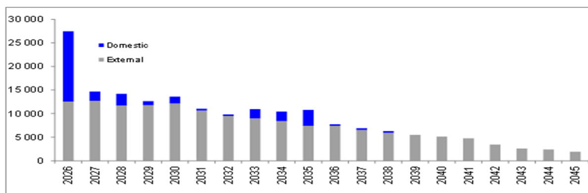
Graphique 4 : Profil de remboursement de la dette projeté à fin 2025 (En millions de USD)
